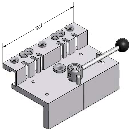
Bohrlehre Blendrahmen Bautiefe 70
