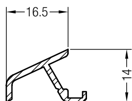
Wetterschenkel 14 Bautiefe 70
