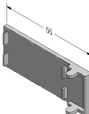
Abdeckkappe Schwellenhalter Bodenschwelle universal Bautiefe 70
