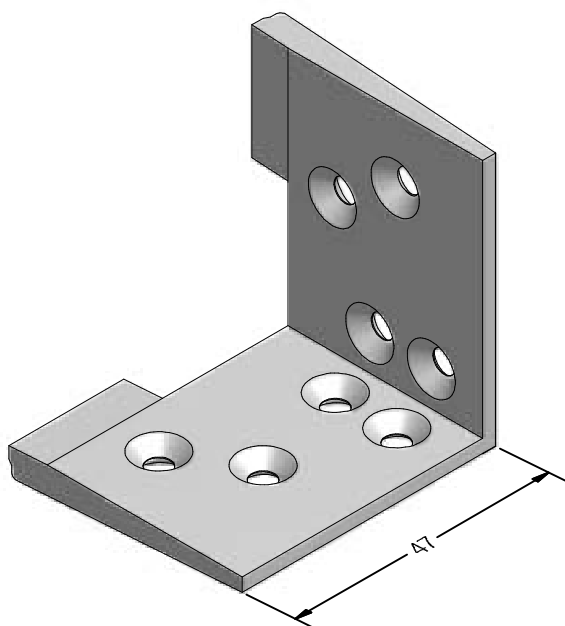
Sprossenwinkel Bautiefe 70
