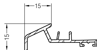
Wetterschenkel 15 Bautiefe 70
