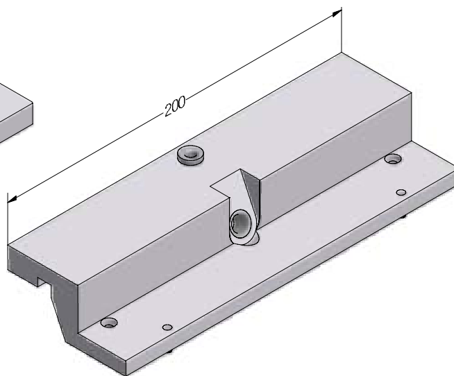
Bohrlehre Belüftung Vorkammern
