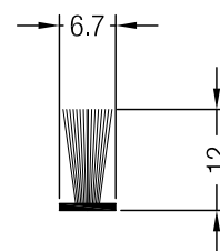
Bürstendichtung 6,7 x 12
