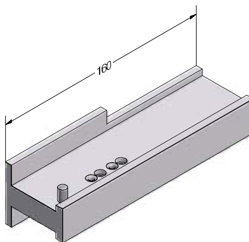
Bohrlehre Pfosten/Sprosse Bautiefe 70
