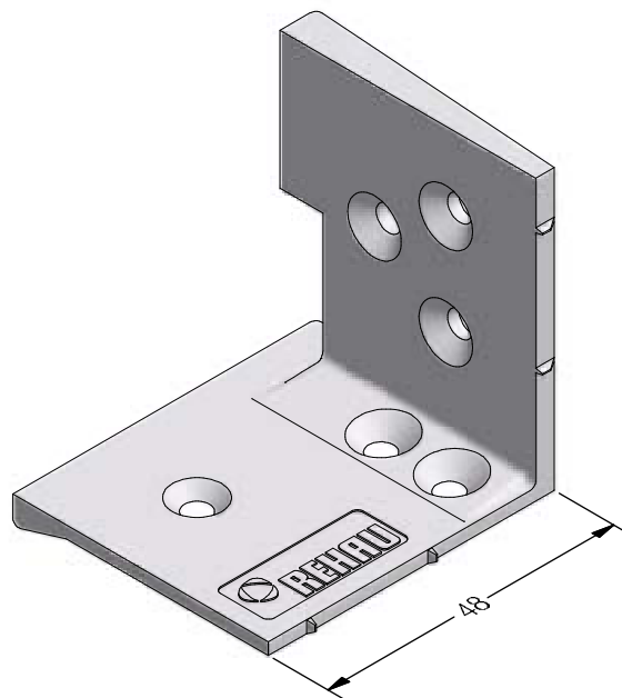
Sprossenwinkel für Flügel Z 54
