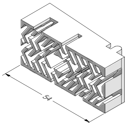
Windstopp für Bodenschwelle universal Bautiefe 70
